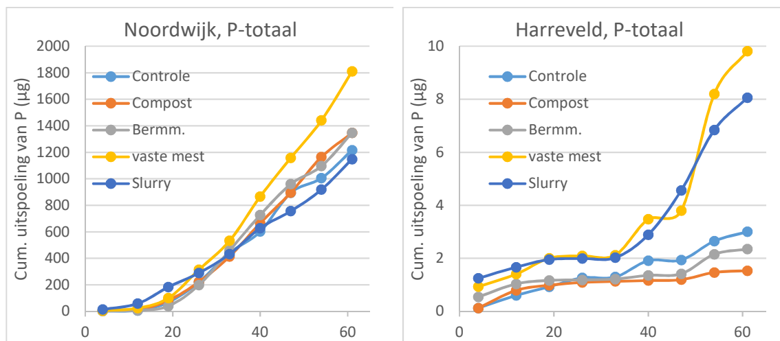
Figuur 4-6 Cumulatieve hoeveelheid P-totaal in het effluent (concentratie x water volume effluent) in de kolommen met Noordwijk grond (links) en met Harreveld grond (rechts).
