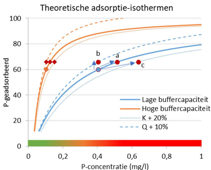
Figuur 1. Twee theoretische adsorptie-isothermen; één met een lage buffercapaciteit (blauwe lijn) en één met een hoge buffercapaciteit bij lage P-concentratie (oranje lijn). Naast deze doorgetrokken lijnen zijn ook de situaties weergegeven wanneer het adsorptiemaximum wordt verhoogd met 10% (gestreepte lijnen) en wanneer de sorptieconstante met 20% wordt verlaagd (gestippelde lijnen). De gekleurde balk geeft een inschatting van het risico op P-emissie naar het watersysteem.
