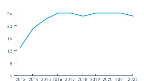
Productie groen gas door afvalsector (in miljoen m 3 )
